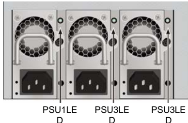
图 20: Vess A2600 电源上的 LED 指示灯
