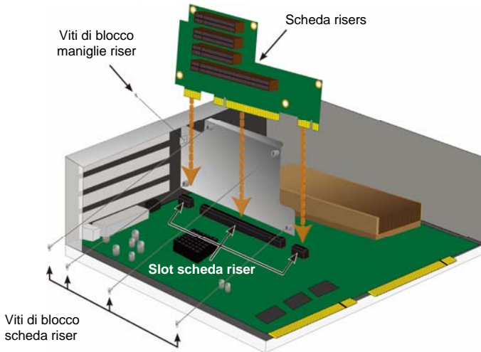
Figura 33: Montare maniglia e inserire scheda raiser
