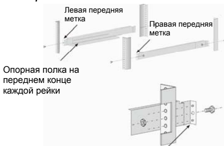
Рисунок 6: Монтаж реек в стойке
