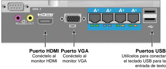
Ilustración 15: Conexiones del monitor de vídeo y los puertos USB del Vess A2600
