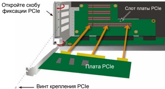
Рисунок 34: Установка платы PCIe
