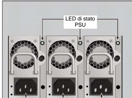
Figura 17: Vess A2600 pannello posteriore N+1 connessioni d'alimentazione
