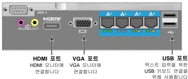
그림 15: Vess A2600 비디오 모니터 연결 및 USB 포트
