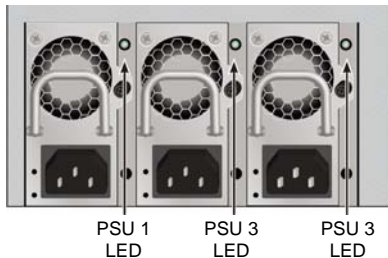
그림 20: Vess A2600의 파워 서플라이 LED
