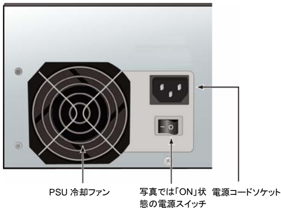
図 16: Vess A2600s 後部パネル電源接続
