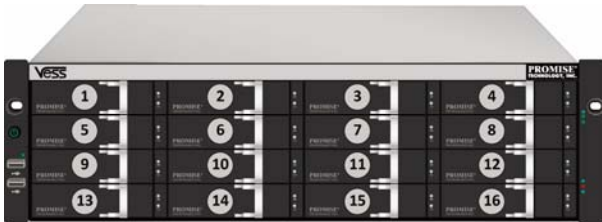
图 11: A2600 的硬盘槽编号
