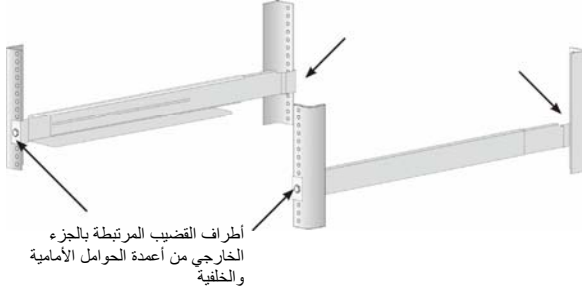
الشكل 7: أطراف القضيبيب المرتبطة بالجزء الخارجي من كل عمود
