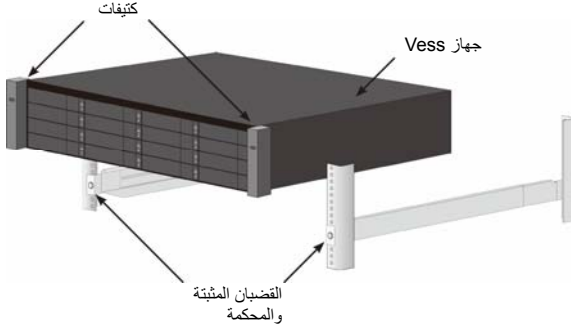
الشكل 8: وضع الجهاز Vess على قضيبيب الحامل
