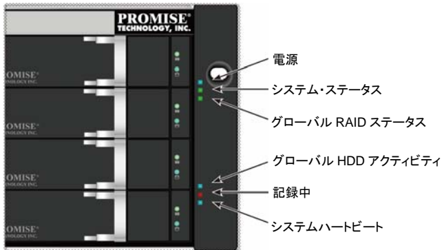
図 19: 右側ブラケット上の Vess フロントパネル LED ディスプレイ
