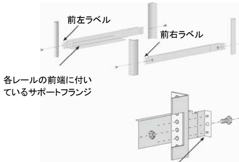
図 6: ラックへのレールの取り付け
