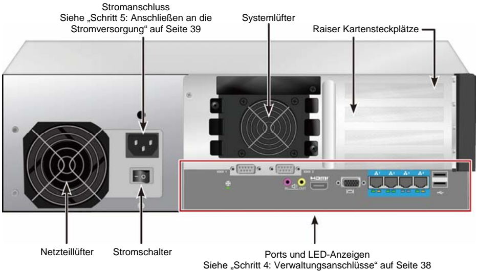
Abbildung 2: Vess A2600s-rückansicht
