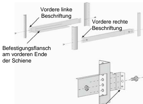
Abbildung 6: Installation der schienen in das rack
