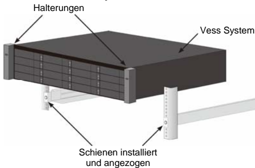
Abbildung 8: Platzieren des Vess systems auf den rack-schienen
