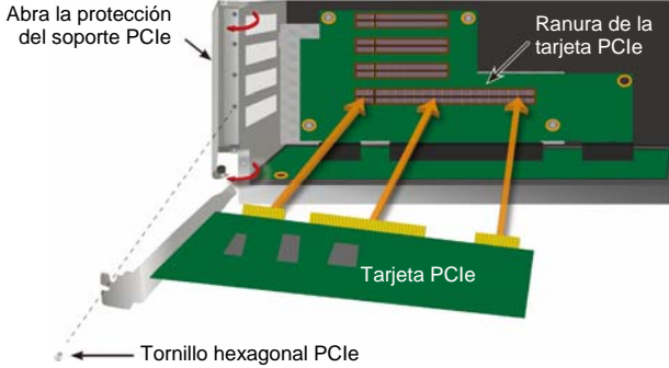
Ilustración 34: Inserte la tarjeta PCIe
