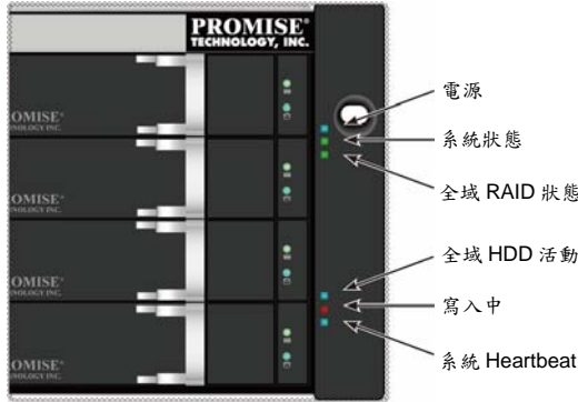
圖 19：右側支架上的 Vess 前方面板 LED 顯示
