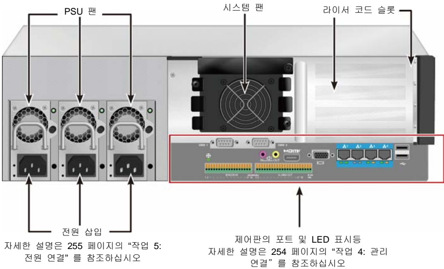
그림 5: Vess A2600 및 레일 브라켓과 팬들
