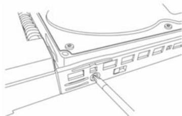
그림 13: 디스크 트레이에 HDD 마운트 하기
